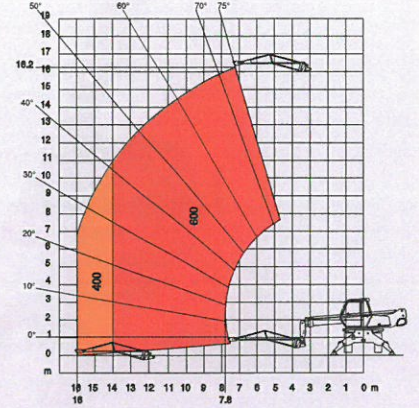
ROTAZIONE SU STABILIZZATORI CON CESTELLO ORH STANDARD 2,25/4 m
