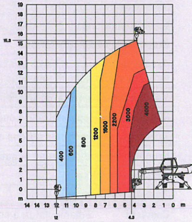
ROTAZIONE SU STABILIZZATORI CON ARGANO 4 T
