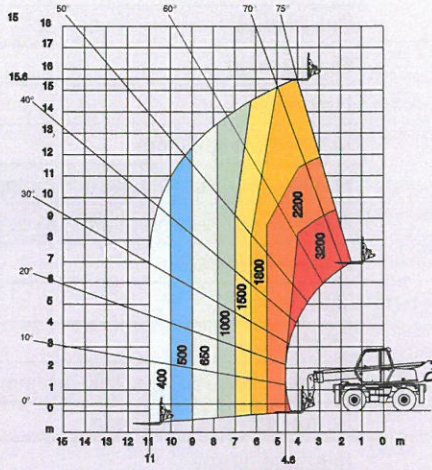
ROTAZIONE SU STABILIZZATORI CON ARGANO 4 T
