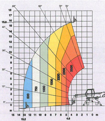
ROTAZIONE SU GOMME CON FORCHE
