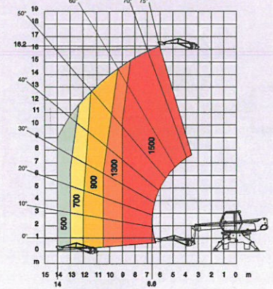
ROTAZIONE SU STABILIZZATORI CON BRACCETTO P 1500
