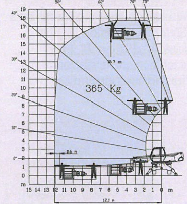
ROTAZIONE SU STABILIZZATORI CON CESTELLO ORH STANDARD 2,25/4 m
