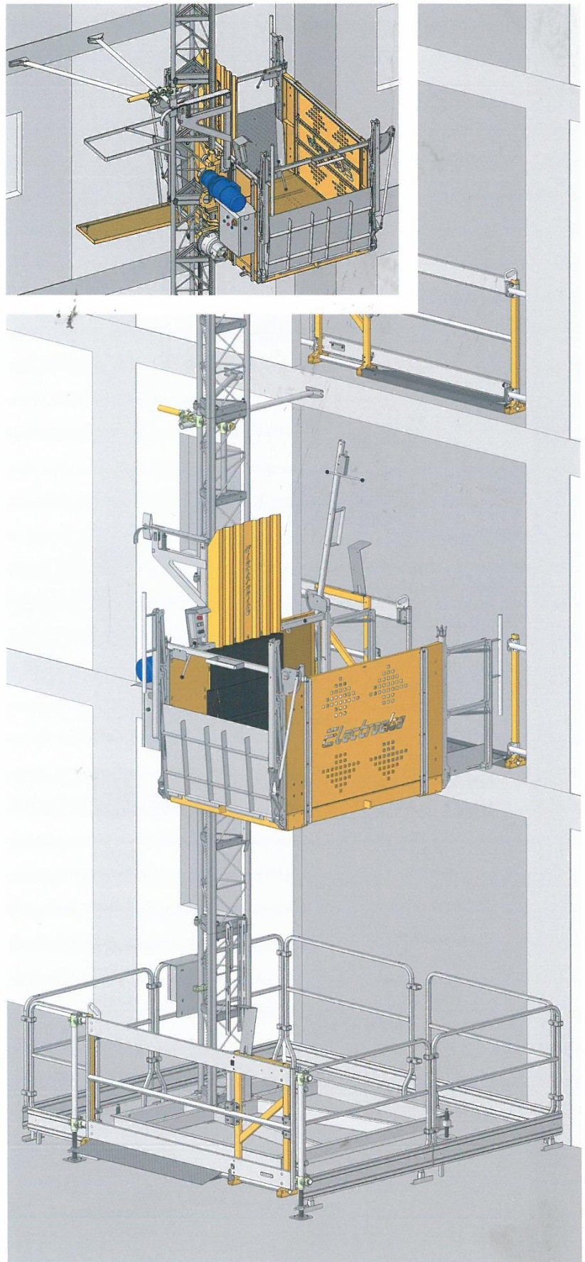
Configurazioni d'accesso possibili Possible access configurations
