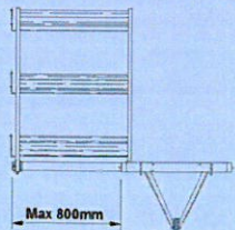
Stabilizzatori rimovibili Removable outriggers
