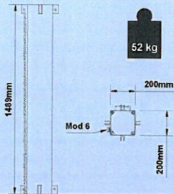
Dettagli moduli ponte Deck module details
