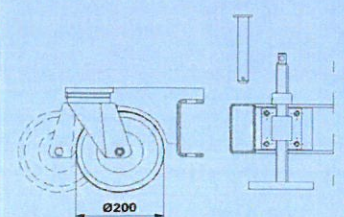
Ruote pivotanti rimovibili Removable pivoting wheels
